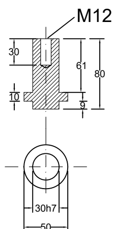
Perno forcella ruota pz 2
